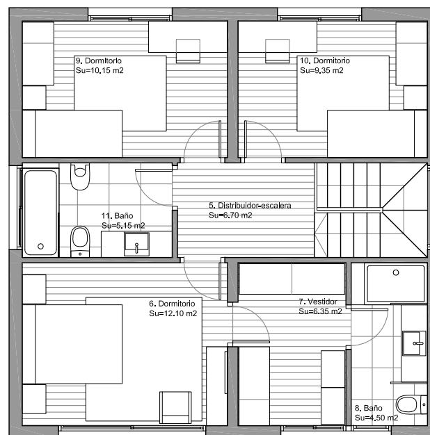
PLANTA PRIMERA ESC. 1/100
