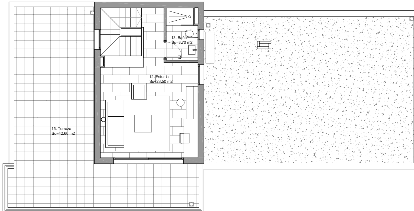
PLANTA PRIMERA ESC. 1/100
