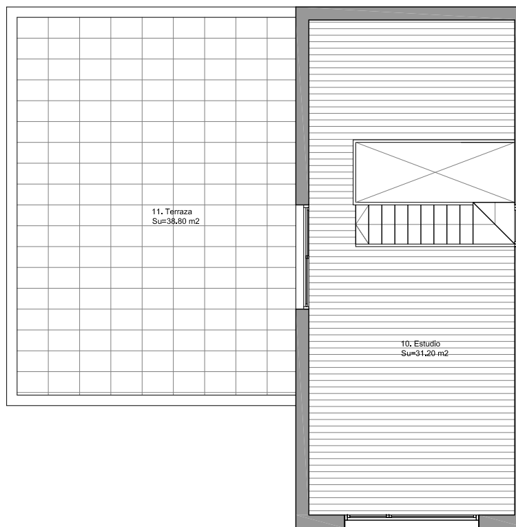
PLANTA PRIMERA ESC. 1/100
