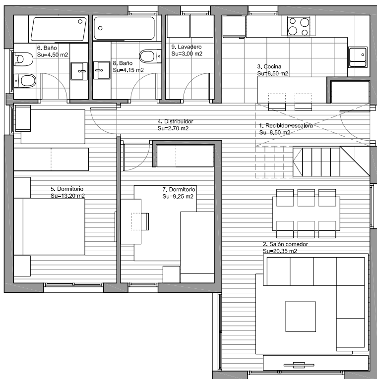
PLANTA BAJA ESC. 1/100
