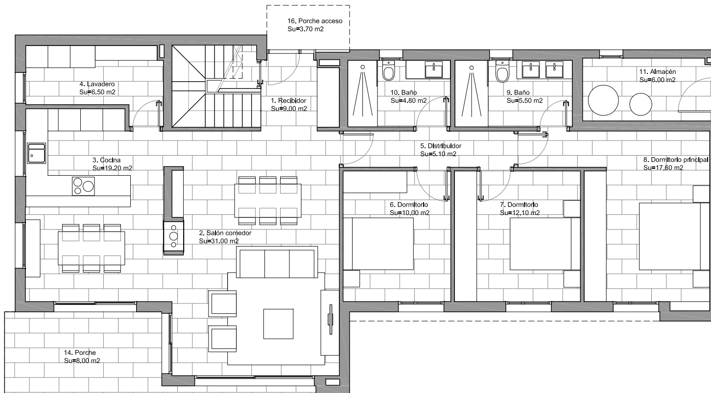
PLANTA BAJA ESC. 1/100
