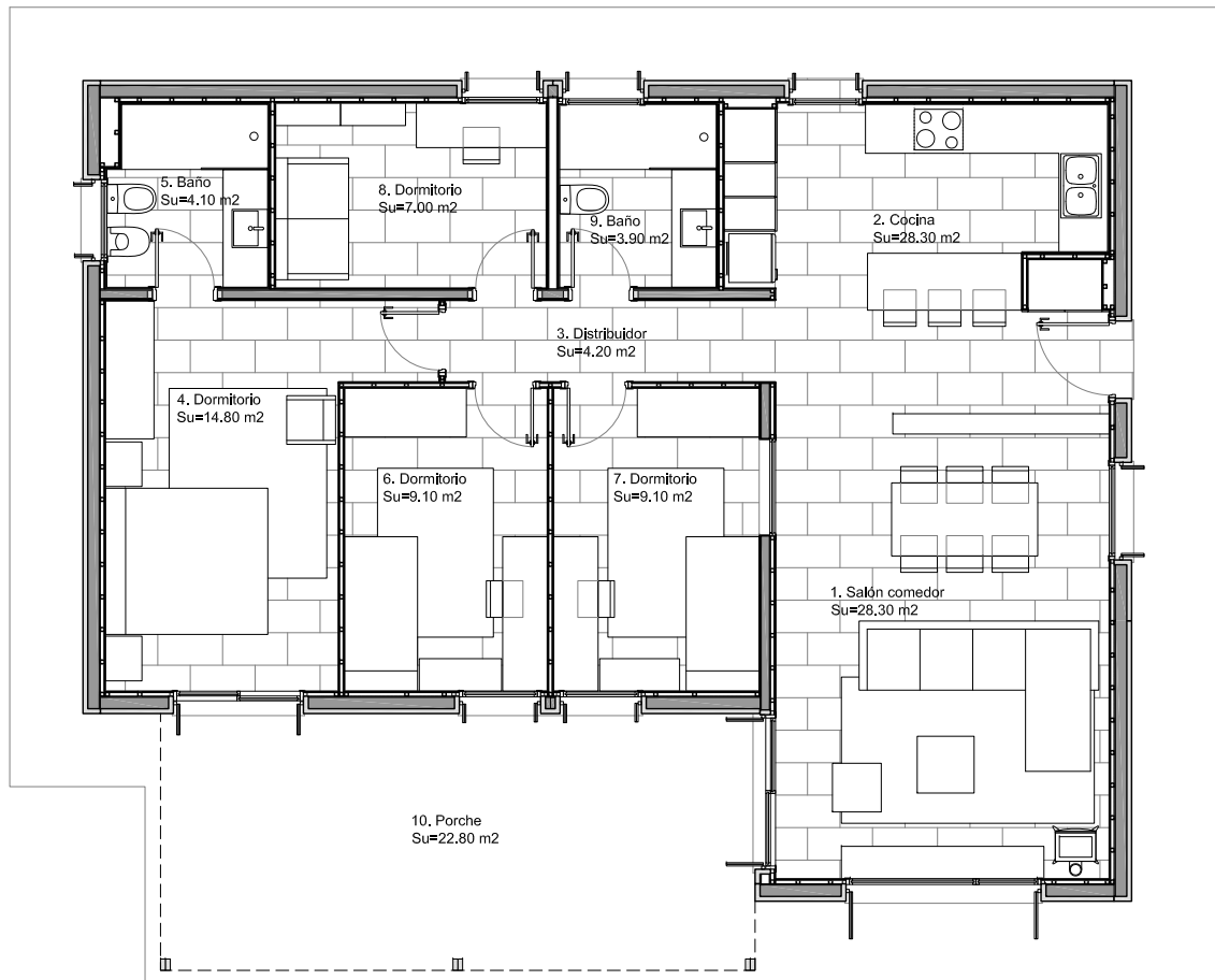
PLANTA ESC. 1/100
