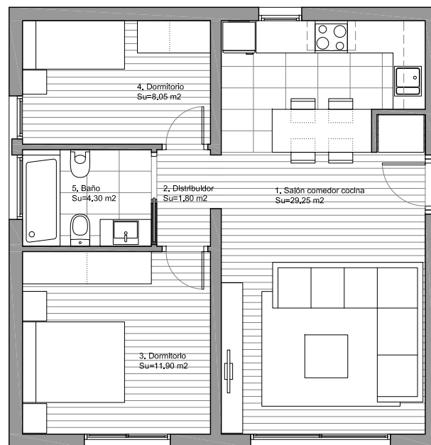
PLANTA ESC. 1/100
