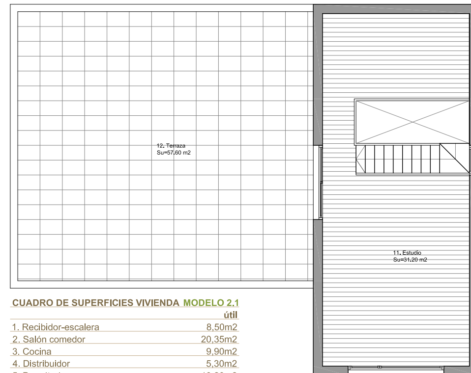
PLANTA PRIMERA ESC. 1/100
