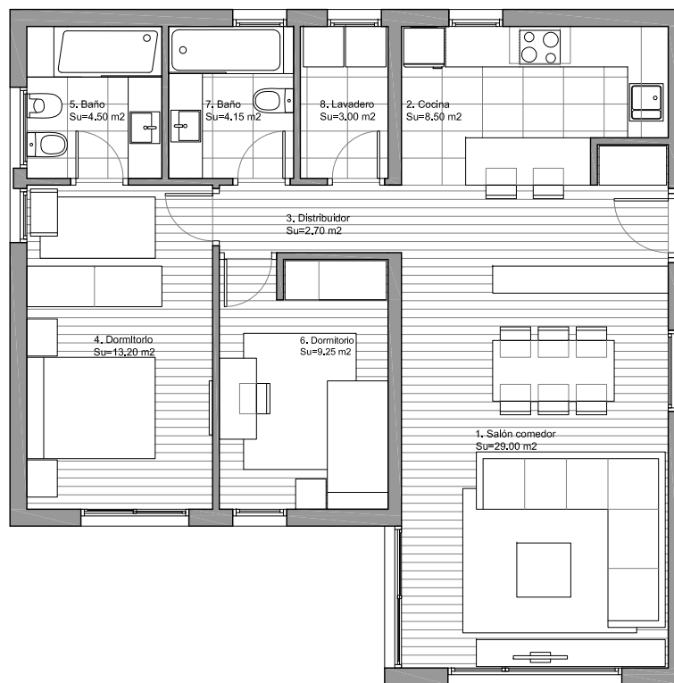
PLANTA ESC. 1/100
